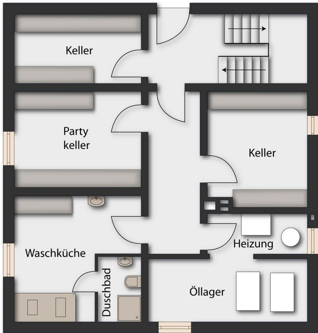
Grundriss KG
